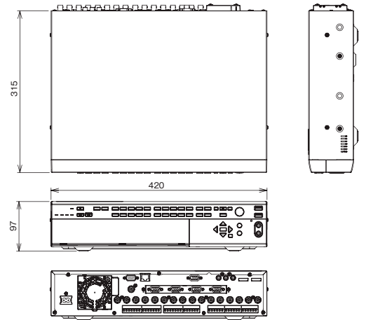
寸法図
