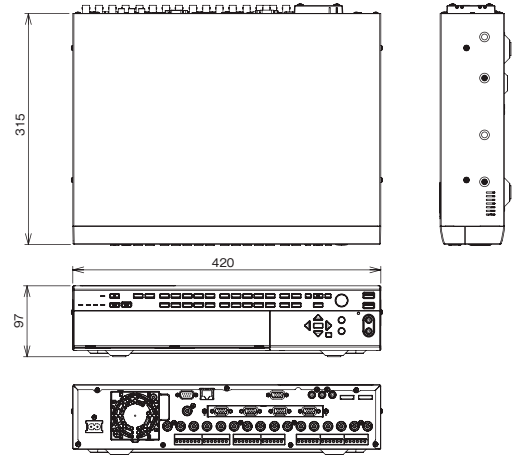
寸法図
