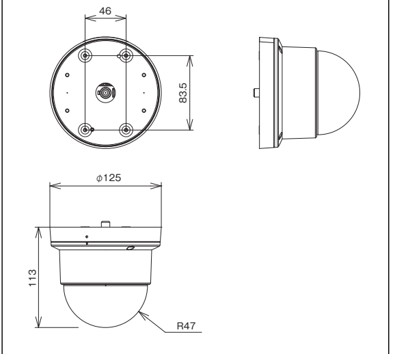
寸法図
