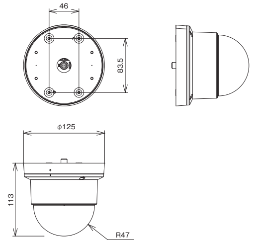
寸法図
