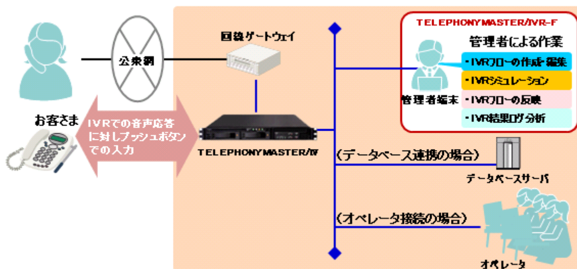
図1 TELEPHONYMASTER/IVと電話音声応答機能のシステム構成(イメージ)
